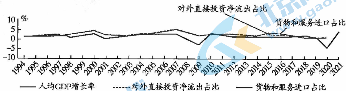
全球主要指标变化情况(1994—2021年)
